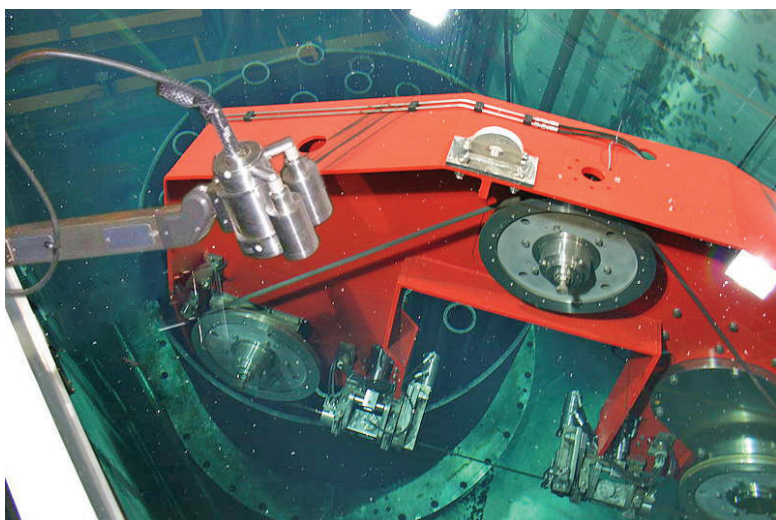
Caméras tolérantes aux rayonnements utilisées pour surveiller la découpe et le démantèlement sous-eau des composants du réacteur
