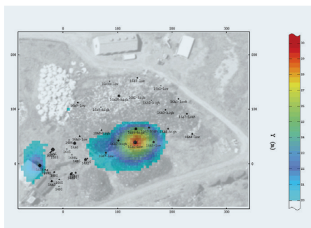
Cartographie de la zone contaminée à ^{235}\text{U}
