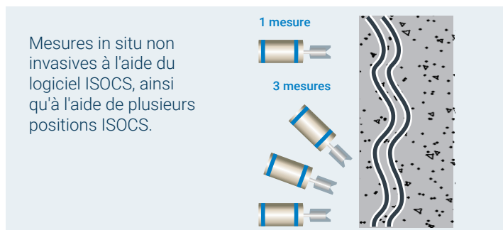
Détermination de la paroi ou de la surface en Bq/cm 2 et détection du profil en profondeur à l'aide d'ISOCS GeHP
