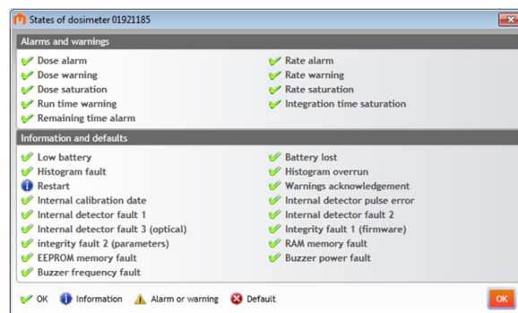
Dosimeter status
